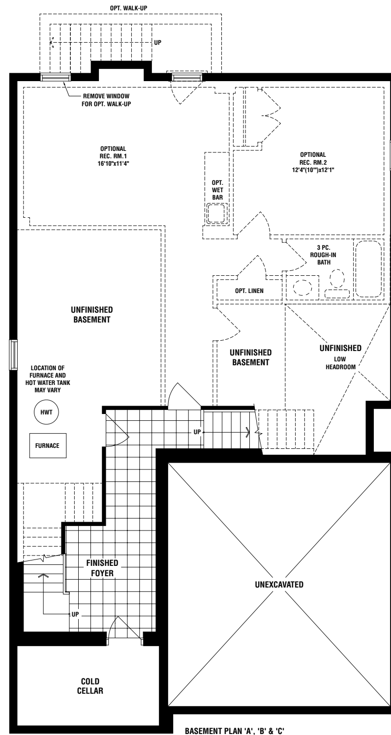
BASEMENT PLAN 'A', 'B' & 'C'
